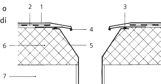
Sezione trasversale di un chiusino installato
