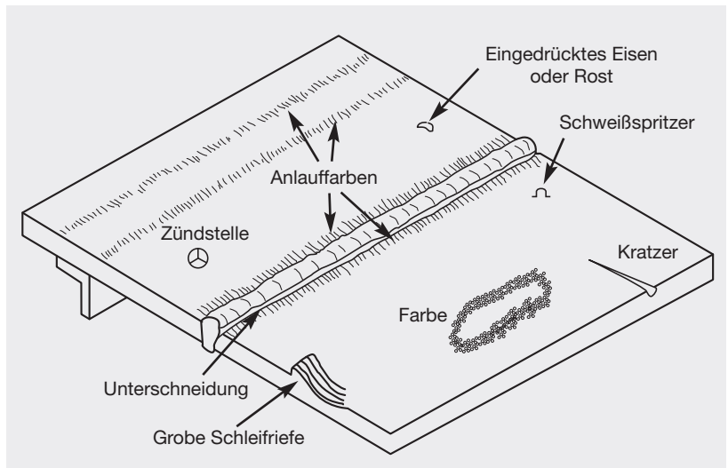
Abbildung 18: Häufig anzutreffende Verarbeitungs- oder Oberflächenfehler (Quelle: Nickel Institute Publication 10 026)
