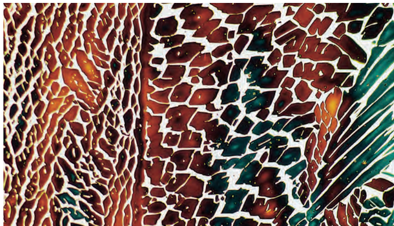
Schliffbild Schweißnaht im Duplexstahl EN 1.4462 (2205) in 500-facher Vergrößerung (Quelle: Lincoln Smitweld bv)
